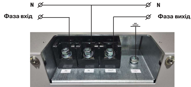
Мал.3. Схема підключення стабілізатора
