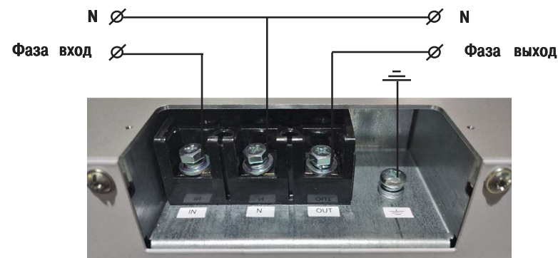
Рис.3. Схема подключения стабилизатора.
