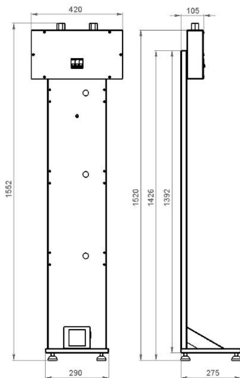
Мал.1. Загальний вигляд Стійки для стабілізаторів 4-14.
