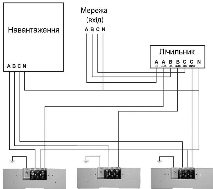
Мал.9. Принципова схема підключення стабілізаторів до трифазної мережі.
