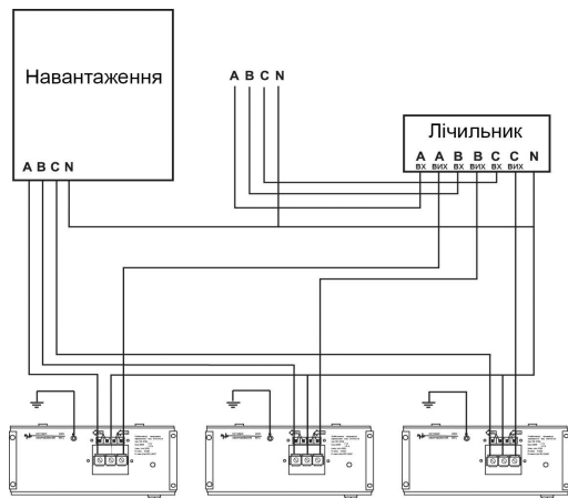
Мал. 10. Принципова схема підключення стабілізаторів до трифазної мережі.
