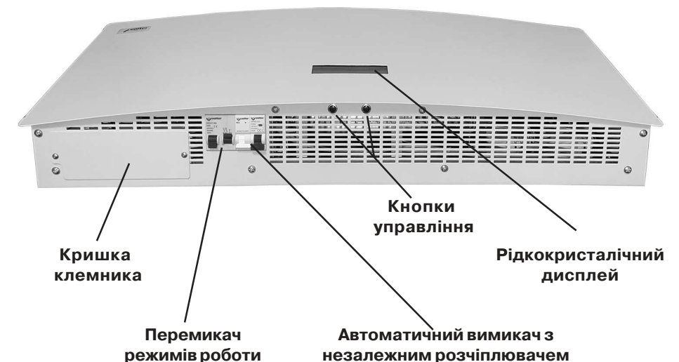
Мал. 1. Стабілізатор напруги Prostor.
