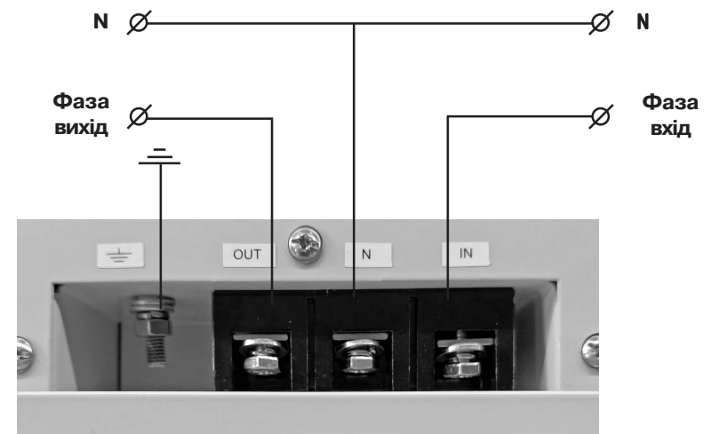
Мал.3. Схема підключення стабілізатора Prostor
