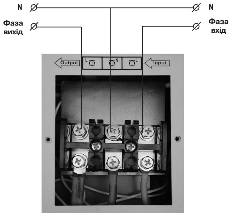
Мал.3. Схема підключення стабілізатора.
