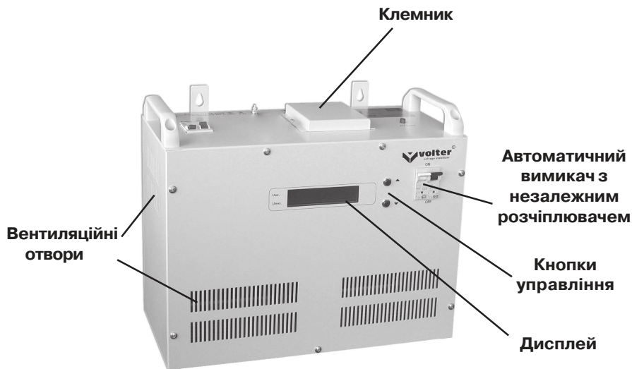
Мал. 1. Стабілізатор напруги СНЗСО-9.
