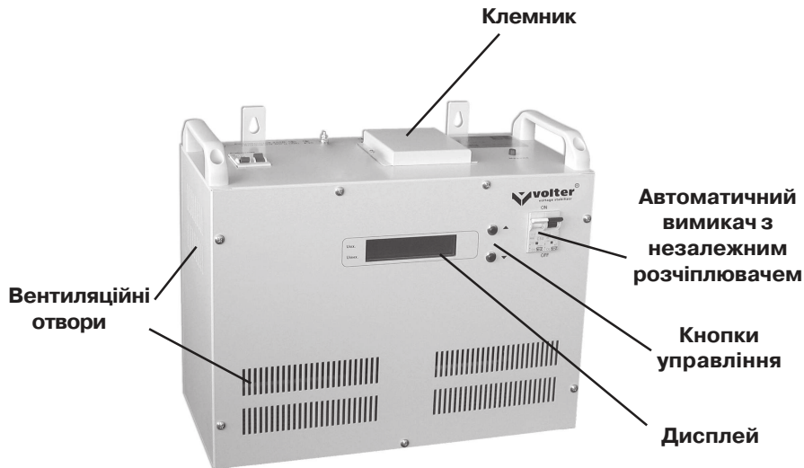
Мал. 1. Стабілізатор напруги СНЗСО-14.
